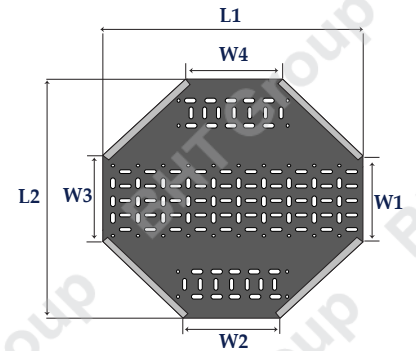
Co chữ thập - Horizontal cross
