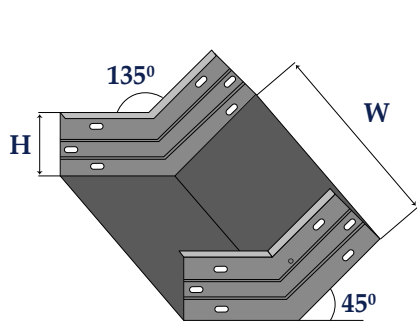
Co lên 45° - Internal riser 45°
