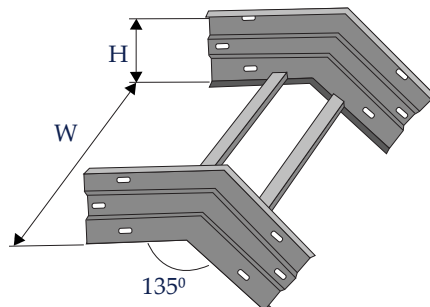
Co xuống 45° - External riser 45°
