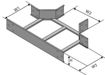
Co chữ T Horizontal T
