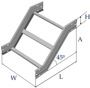
Co Z đứng - Internal riser 45°
