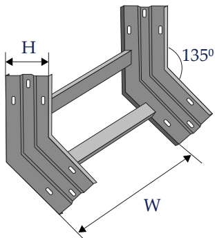
Co lên 45° - Internal riser 45°
