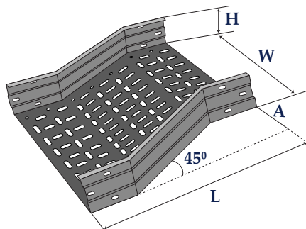
Co Z ngang phải - Right horizontal Z
