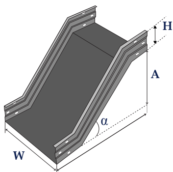
Co Z đứng - Vertical Z
