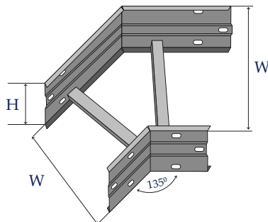
Co ngang 45° - Horizontal elbow 45°
