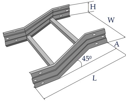
Co Z ngang phải - Right horizontal Z
