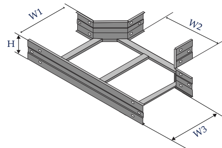
Co chữ T - Horizontal T
