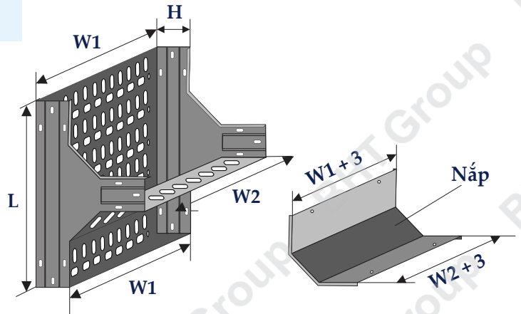
Co T đứng trục dọc - T shaped hinge vertical
