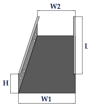
Co giảm trái - Left reducer
