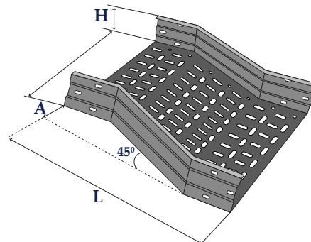
Co Z ngang trái - Left horizontal Z
