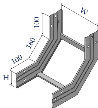
Co lên 90° - Internal riser 90°
