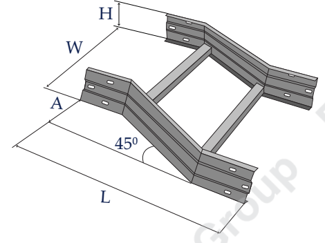
Co Z ngang trái - Left horizontal Z
