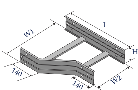
Co giảm phải - Right reducer
