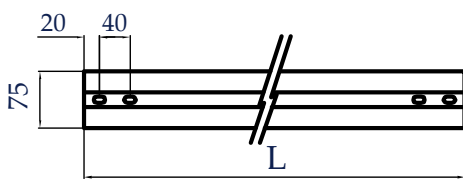
WxH50xL
