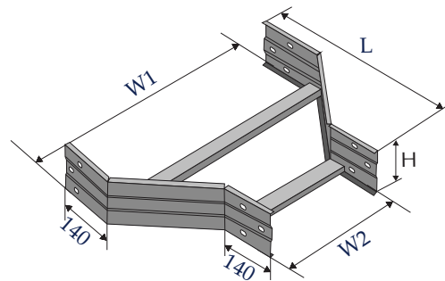
Co giảm giữa - Offset reducer
