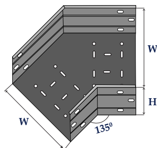
Co ngang 45° - Horizontal elbow 45°
