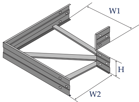
Co ngang 90° - Horizontal elbow 90°
