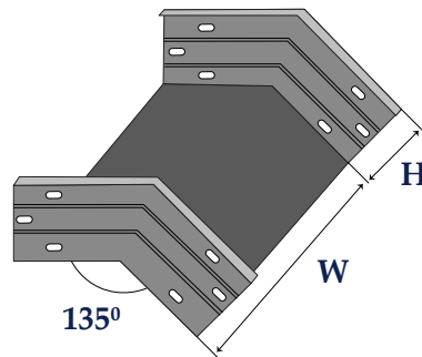
Co xuống 45° - External riser 45°
