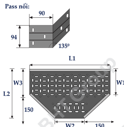
Co chữ T - Horizontal T
