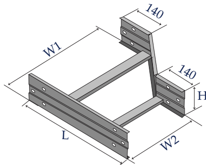
Co giảm trái - Left reducer
