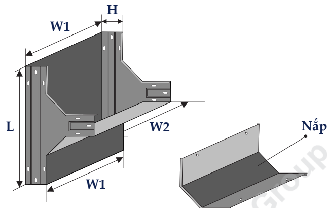
Co T đứng trục dọc - T shaped hinge vertical
