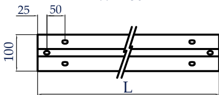
WxH50xL
