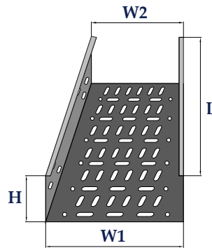
Co giảm trái - Left reducer
