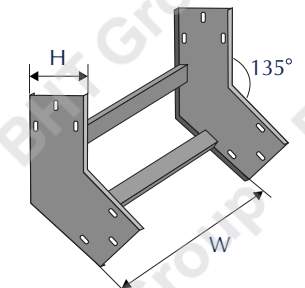
Co lên 45° Internal riser 45°
