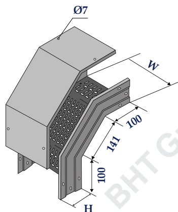
Co xuống 90° - External riser 90°
