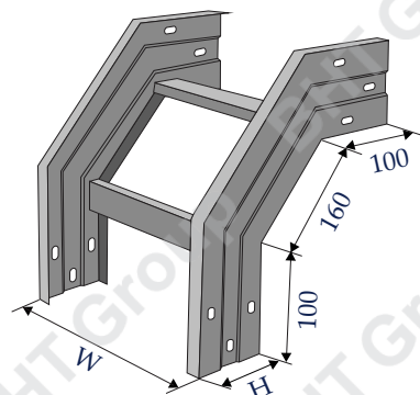
Co xuống 90° - External riser 90°
