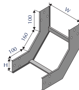
Co lên 90° Internal riser 90°
