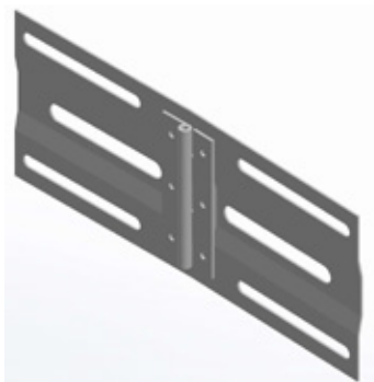
Nối xoay ngang ngoài Connector for outer horizontal hinge
