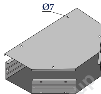
Co chữ T - Horizontal T
