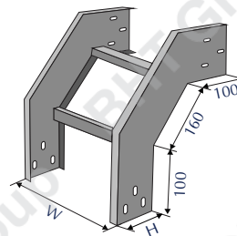
Co xuống 90° External riser 90°
