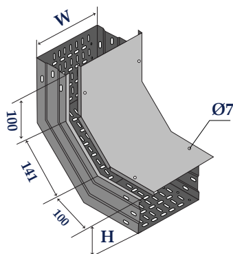
Co lên 90° - Internal riser 90°
