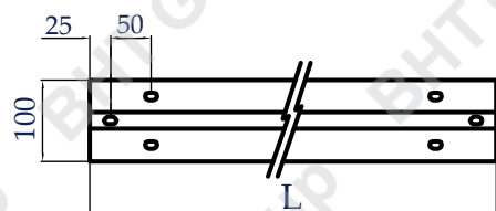
WxH50xL
