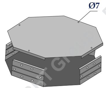
Co chữ thập - Horizontal cross
