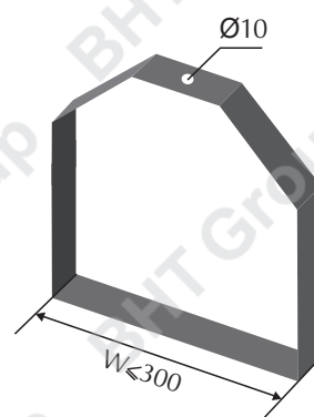
Cùm Treo Máng Cáp Clevirs Hange
