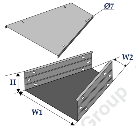
Co giảm giữa - Offset reducer
