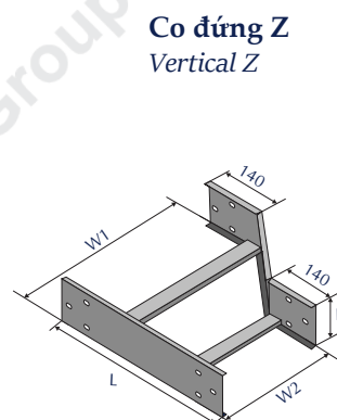
Co giảm trái Left reducer
