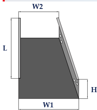
Co giảm phải - Right reducer
