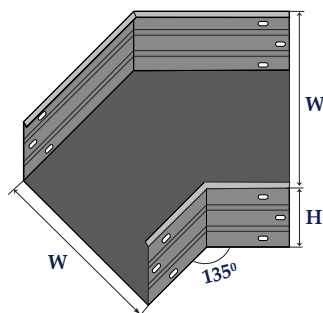
Co ngang 45° - Horizontal elbow 45°
