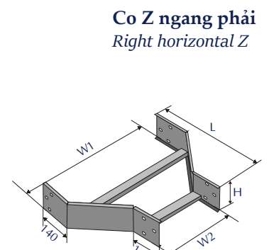
Co giảm giữa Offset reducer
