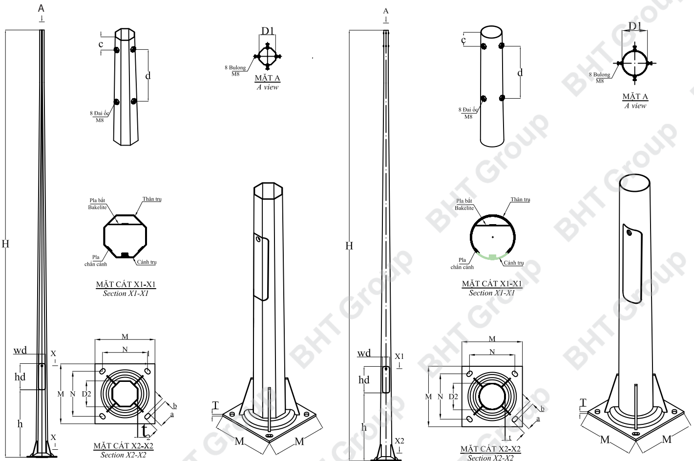
Trụ thép tròn côn / Circular tapered steel poles
