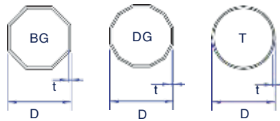
Mặt cắt thân cột Cross section of pole
