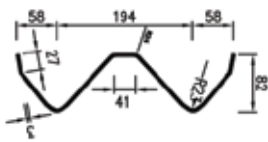
Mặt cắt A-A Cross section A-A
