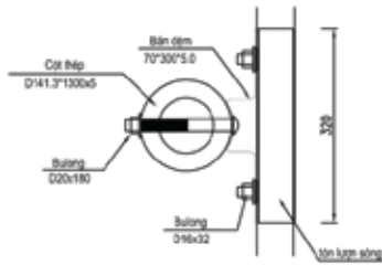
Mặt cắt B-B Cross section B-B
