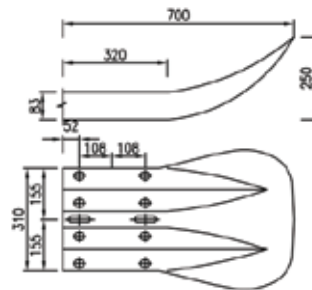
Chi tiết đầu thanh Tôn lượn sóng
